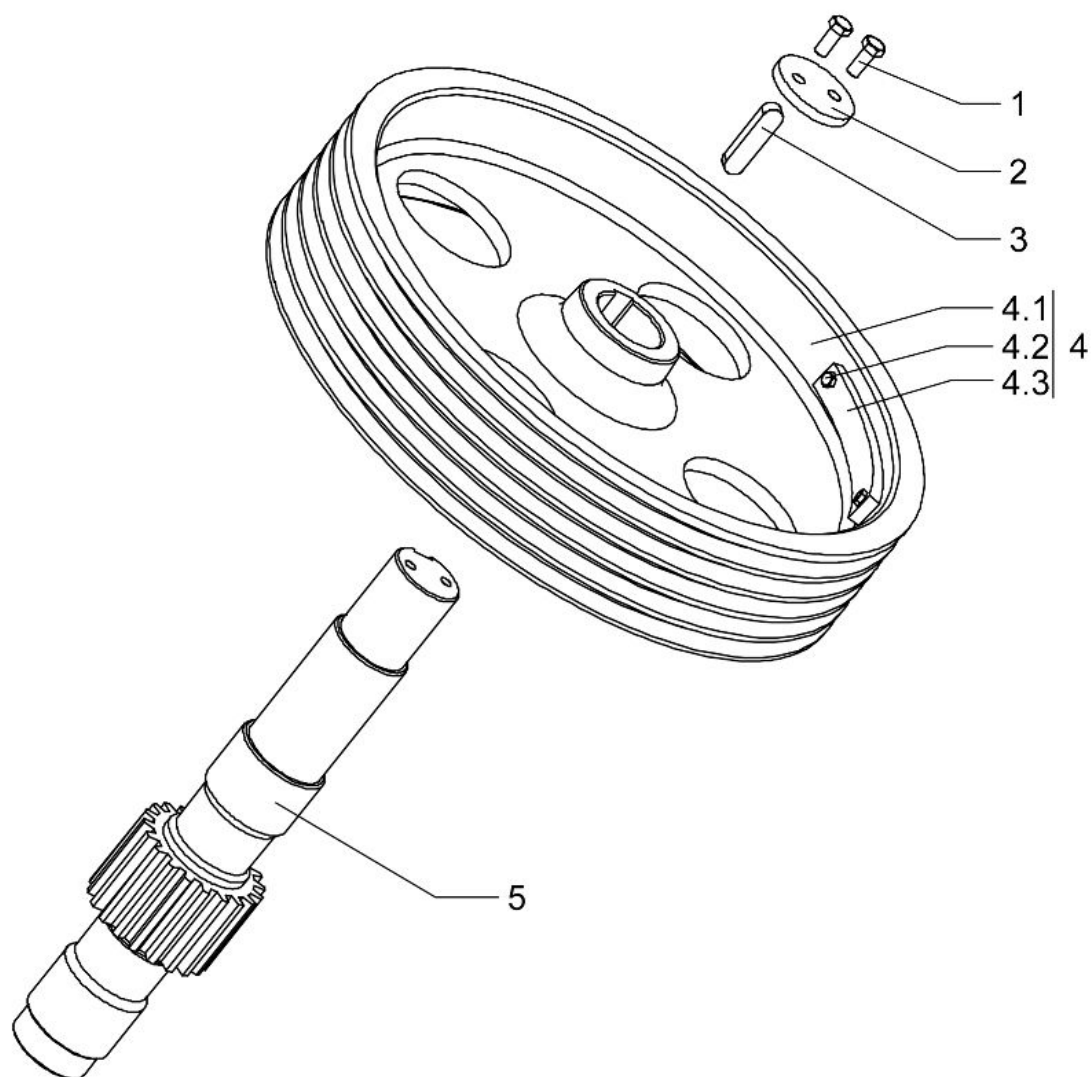
Рис.15. Узел трансмиссионный 01.
