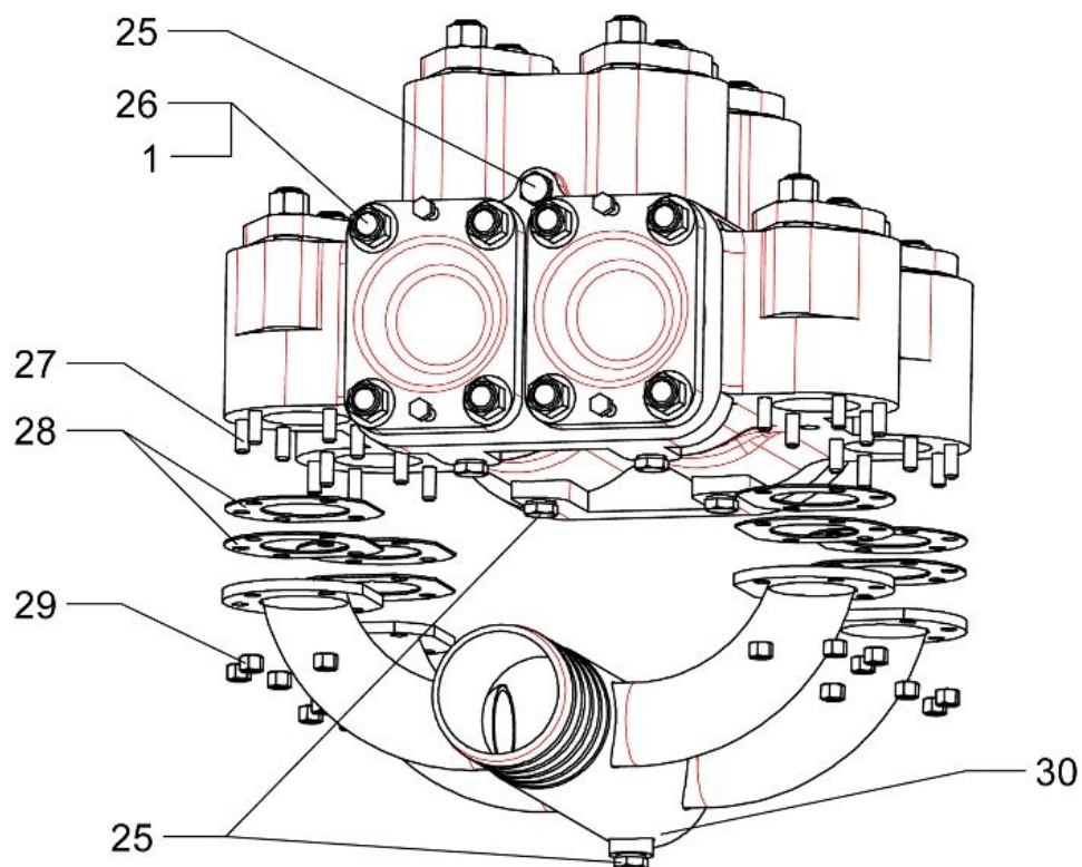
Рис. 6. Блок гидравлический НБ32.02.000. Вид снизу.
