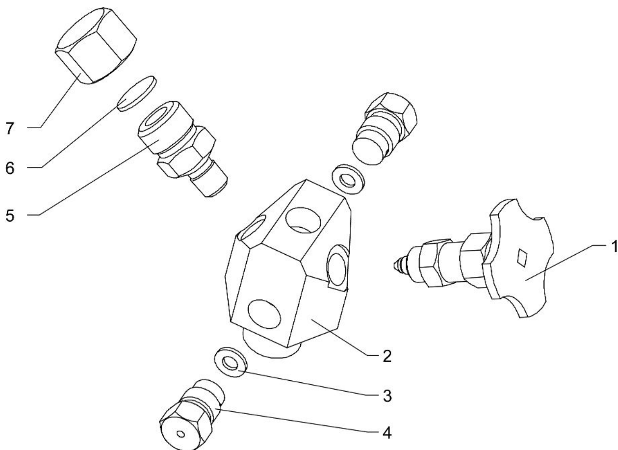
Рис.9. Переходник в сборе КС-10.13.00.000.
