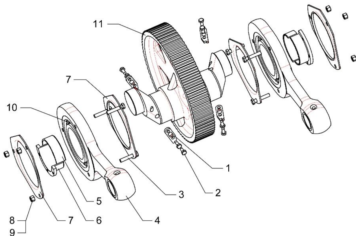
Рис.12. Вал эксцентриковый с шатунами НБ32.01.010.
