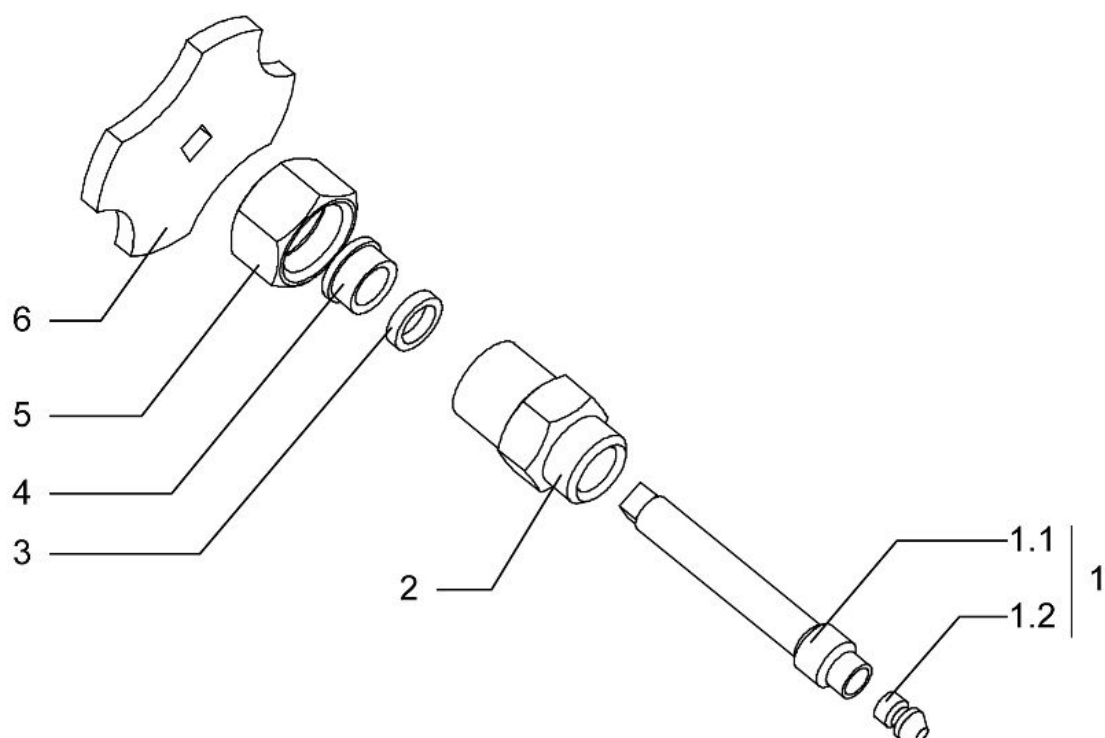
Рис.10. Вентиль игольчатый КС-10.02.00.000.
