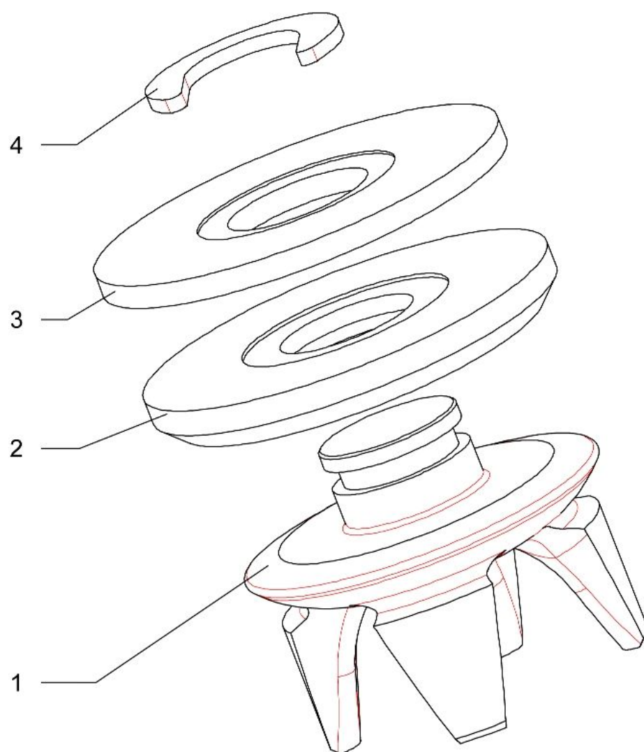
Рис.7. Клапан тарельчатый К2А.01.00.000.
