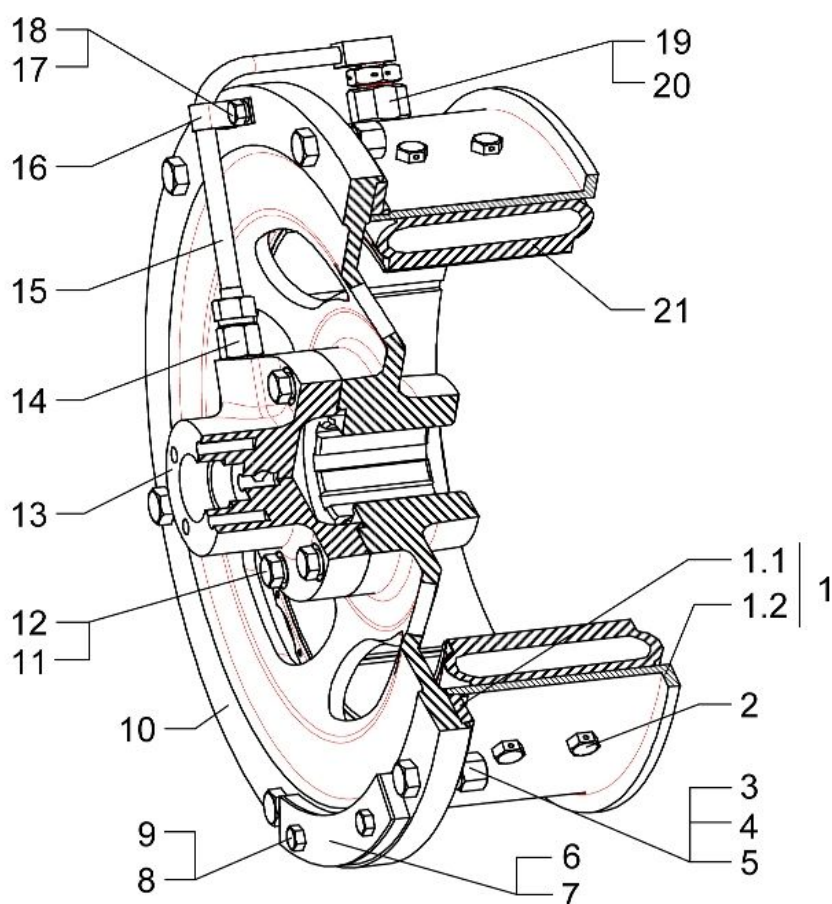
Рис.17. Планшайба НБ40.04.100.
