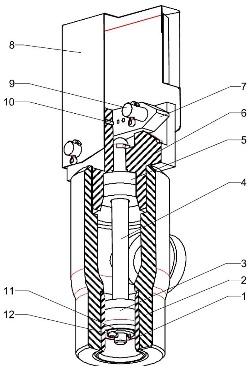
Рис.14. Клапан предохранительный КС-10.12.00.000.
