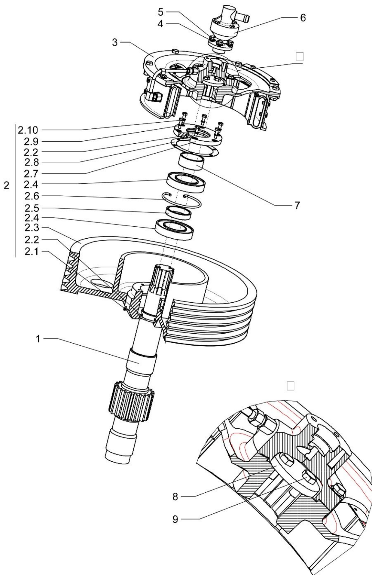
Рис.16. Узел трансмиссионный 03.
