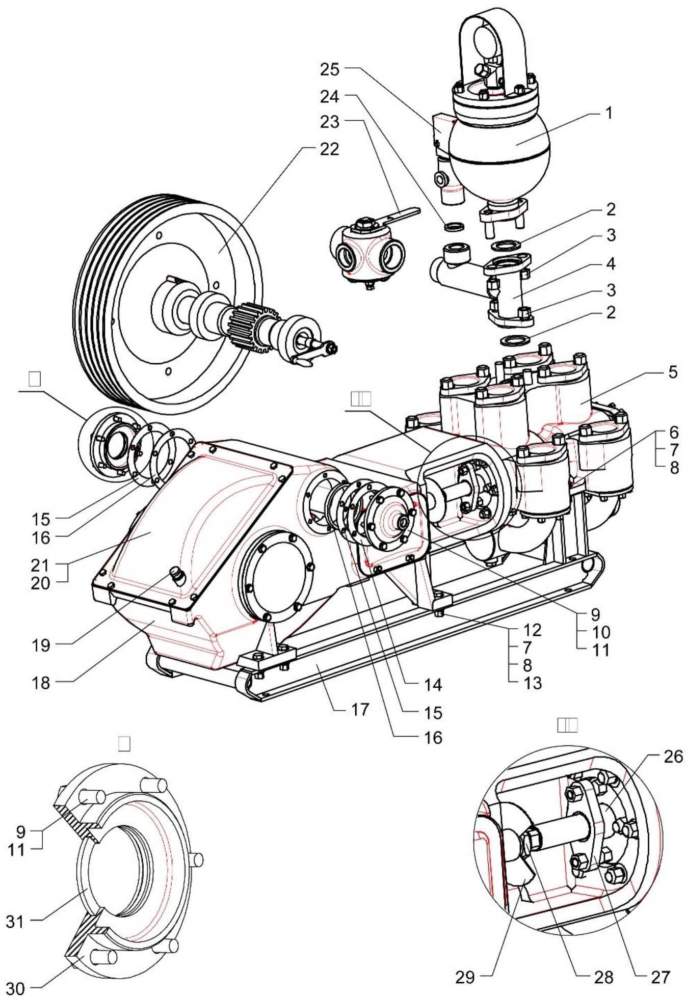
Рис.3. Насос поршневой буровой. Исполнение -05.
