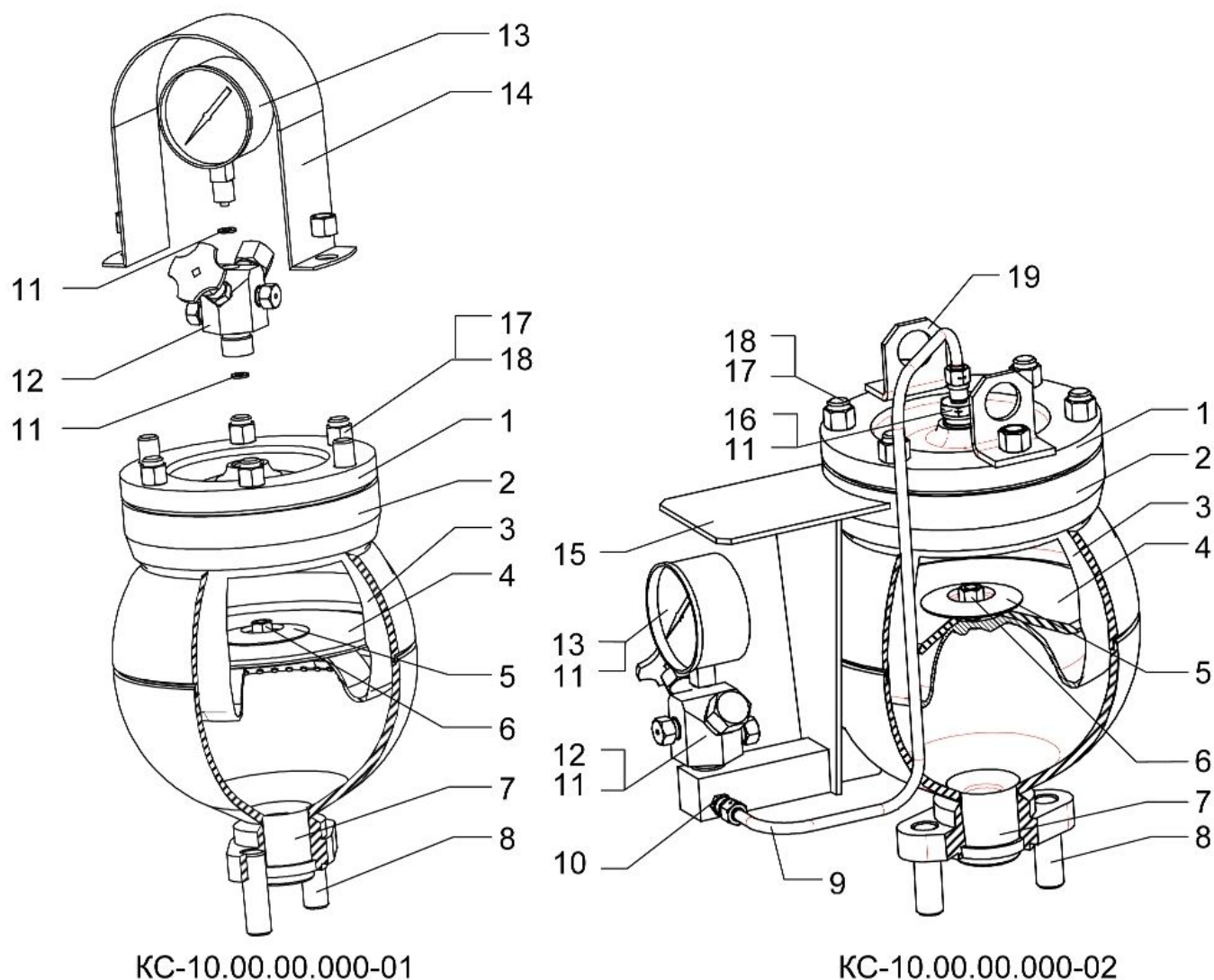
Рис.8. Компенсаторы сферические.
