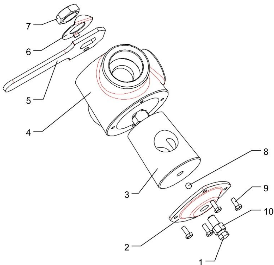
Рис.13. Кран трехходовый НБ40.01.110.
